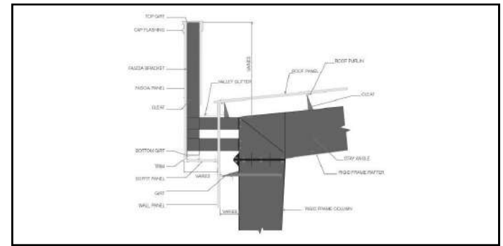
RIGID FRAME COLUMN
